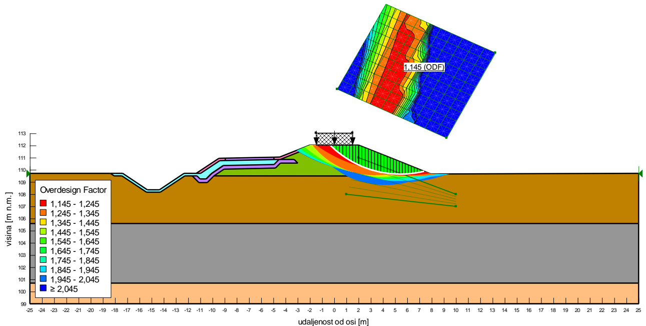
Slika 4.1.32: Situacija 1, uzvodni pokos, drenirano stanje
