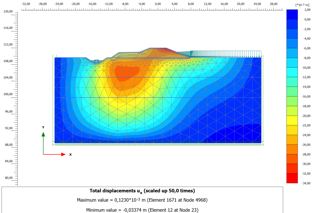
Slika 4.1.72: Raspodjela horizontalnih pomaka za slučaj djelovanja 100 god. velikog vala – situacija 3
