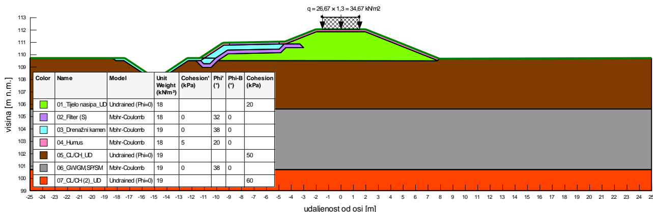
Slika 4.1.28: Geotehnički model nasipa profil 2 i temeljnog tla za provedbu analiza stabilnosti – situacija 1 (nedrenirani parametri)
