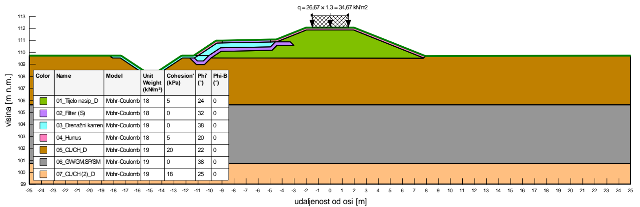
Slika 4.1.49: Geotehnički model nasipa profil 3 i temeljnog tla za provedbu analiza stabilnosti – situacija 1 (drenirani parametri)
