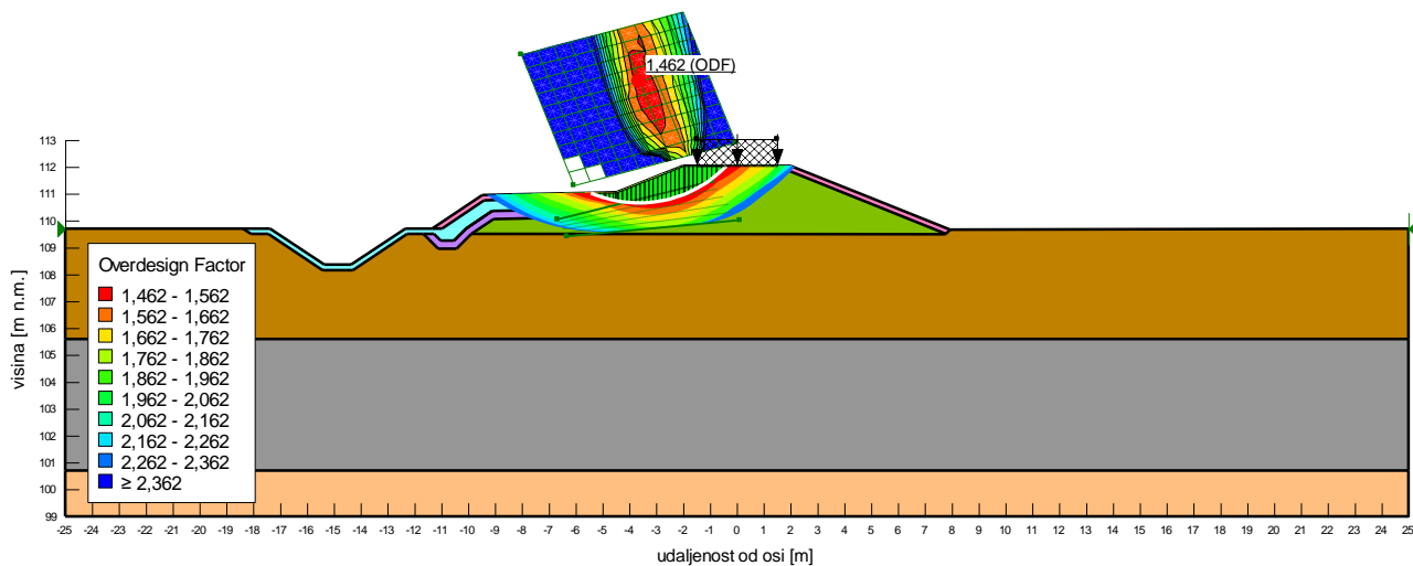
Slika 4.1.15: Situacija 1, nizvodni pokos, drenirano stanje
