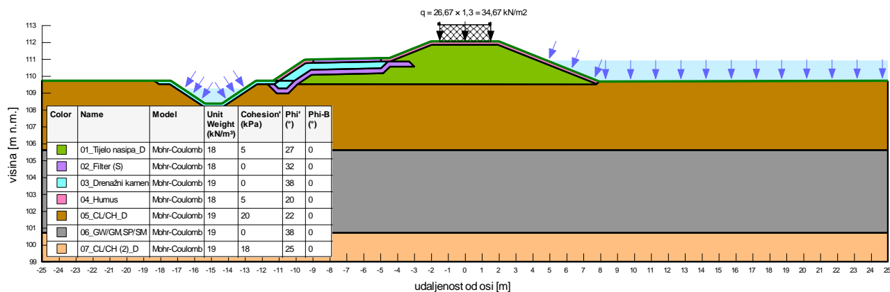
Slika 4.1.19: Geotehnički model nasipa profil 1 i temeljnog tla za provedbu analiza stabilnosti – situacija 3 (drenirani parametri)
