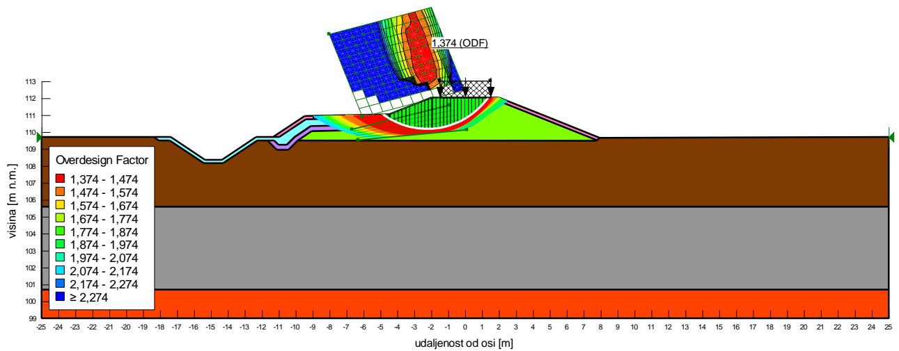
Slika 4.1.31: Situacija 1, nizvodni pokos, nedrenirano stanje
