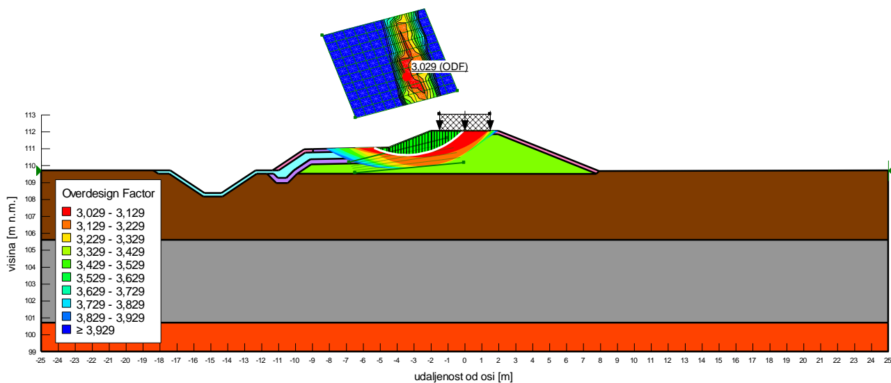
Slika 4.1.13: Situacija 1, nizvodni pokos, nedrenirano stanje
