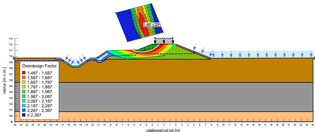
Slika 4.1.21: Situacija 3, nizvodni pokos, drenirano stanje
