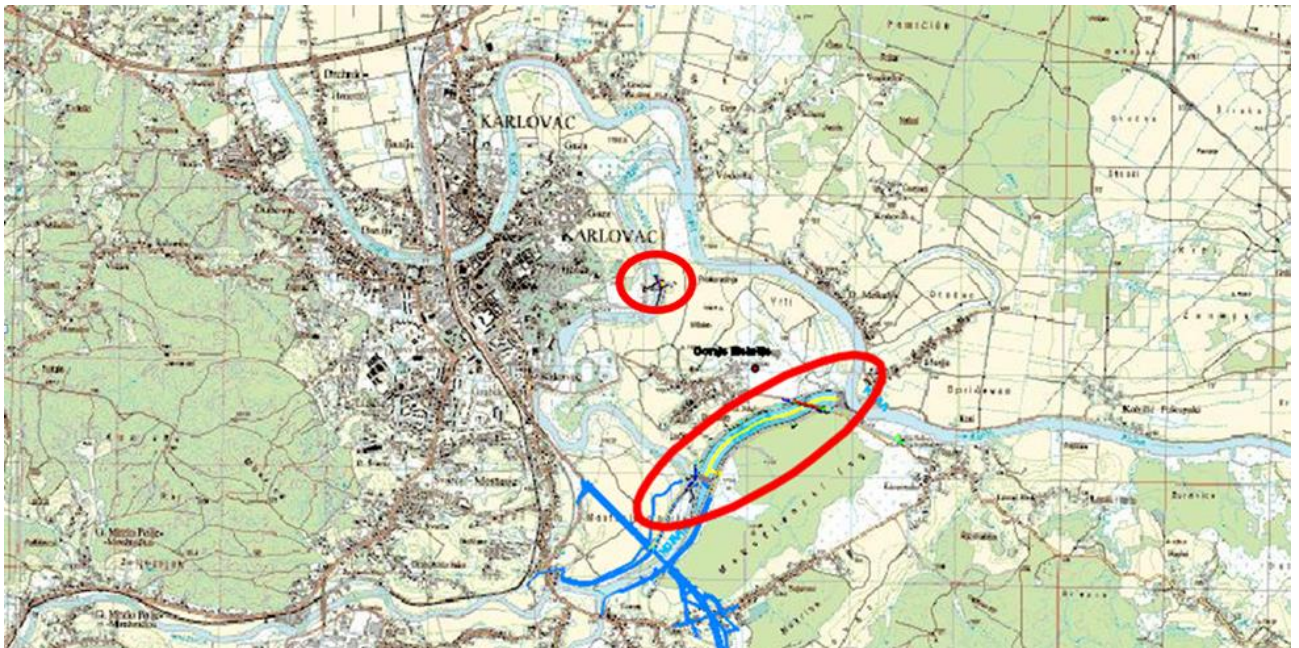
sl. 3.1.2 Lokacija zahvata prokopa s pratećim objektima
