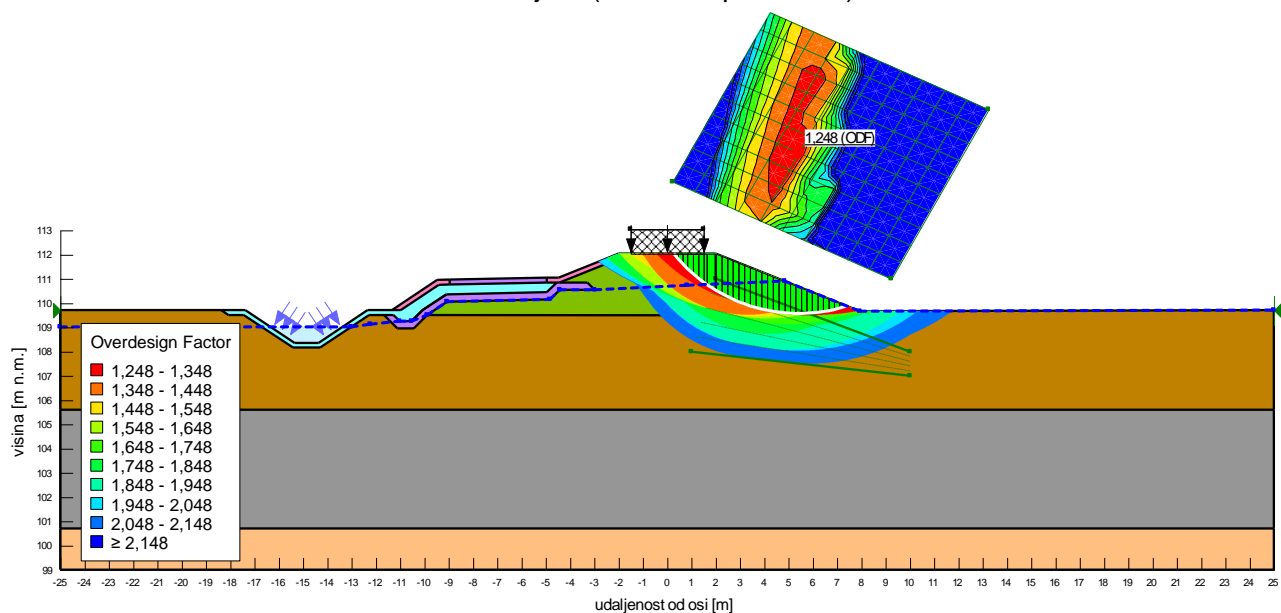
Slika 4.1.26: Situacija 5, uzvodni pokos, drenirano stanje
