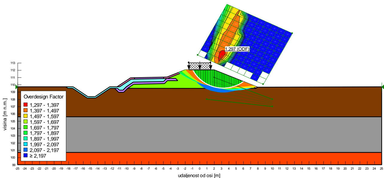
Slika 4.1.30: Situacija 1, uzvodni pokos, nedrenirano stanje
