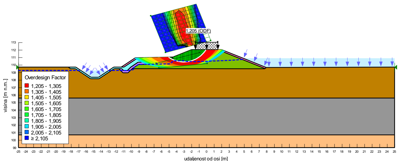
Slika 4.1.39: Situacija 3, nizvodni pokos, drenirano stanje
