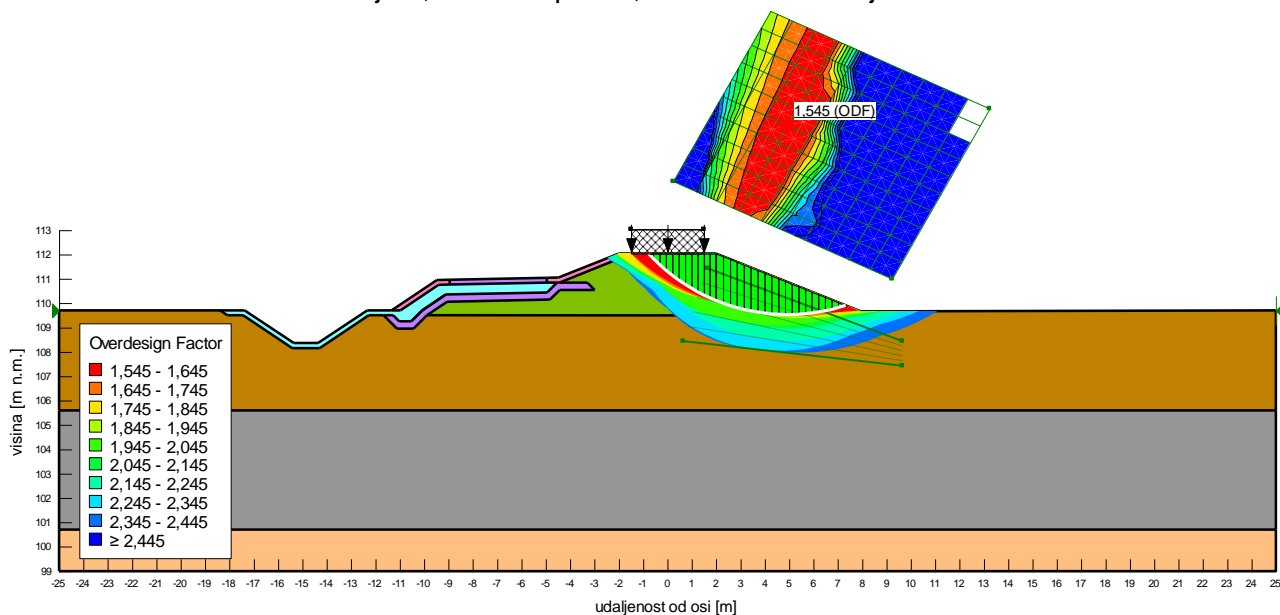
Slika 4.1.14: Situacija 1, uzvodni pokos, drenirano stanje
