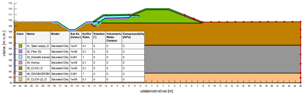
Slika 4.1.1: Geotehnički model nasipa profil 1 i temeljnog tla za provedbu analiza procjeđivanja – situacija
