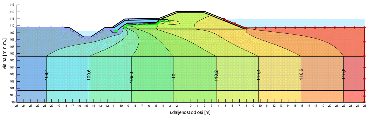
Slika 4.1.2: Hidraulički potencijali za Situaciju 1
