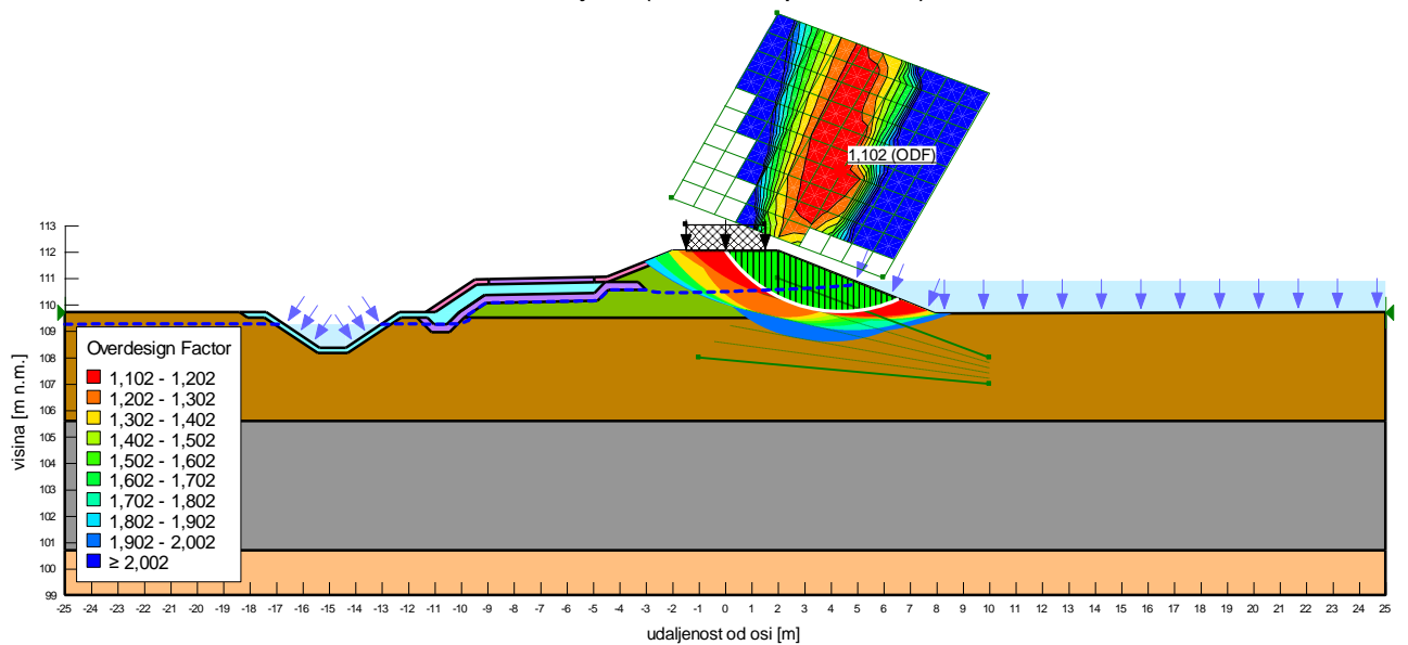
Slika 4.1.38: Situacija 3, uzvodni pokos, drenirano stanje
