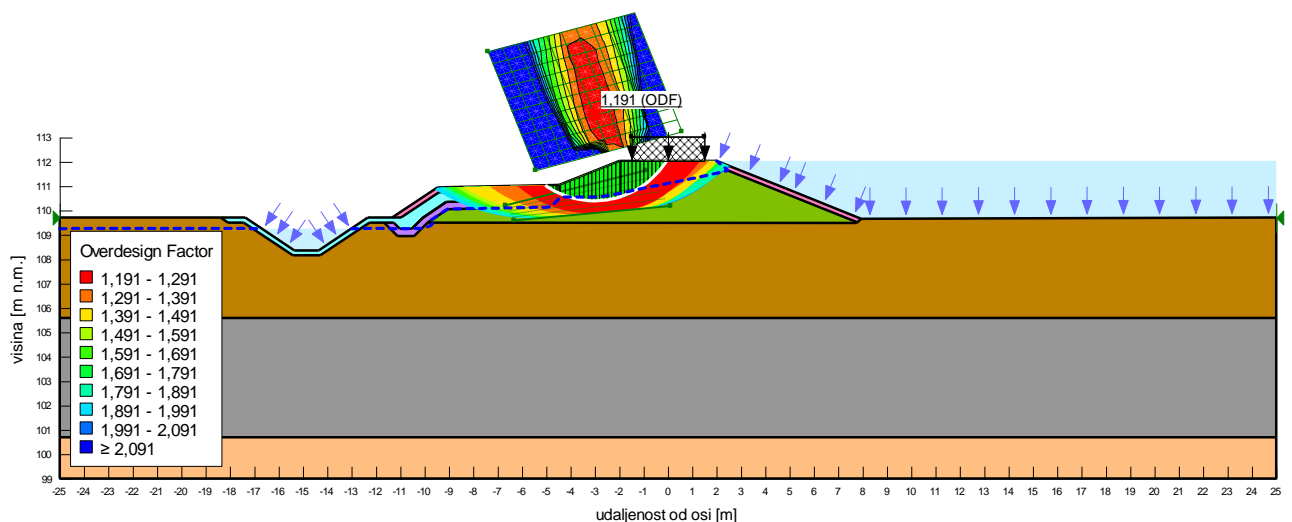
Slika 4.1.42: Situacija 4, nizvodni pokos, drenirano stanje
