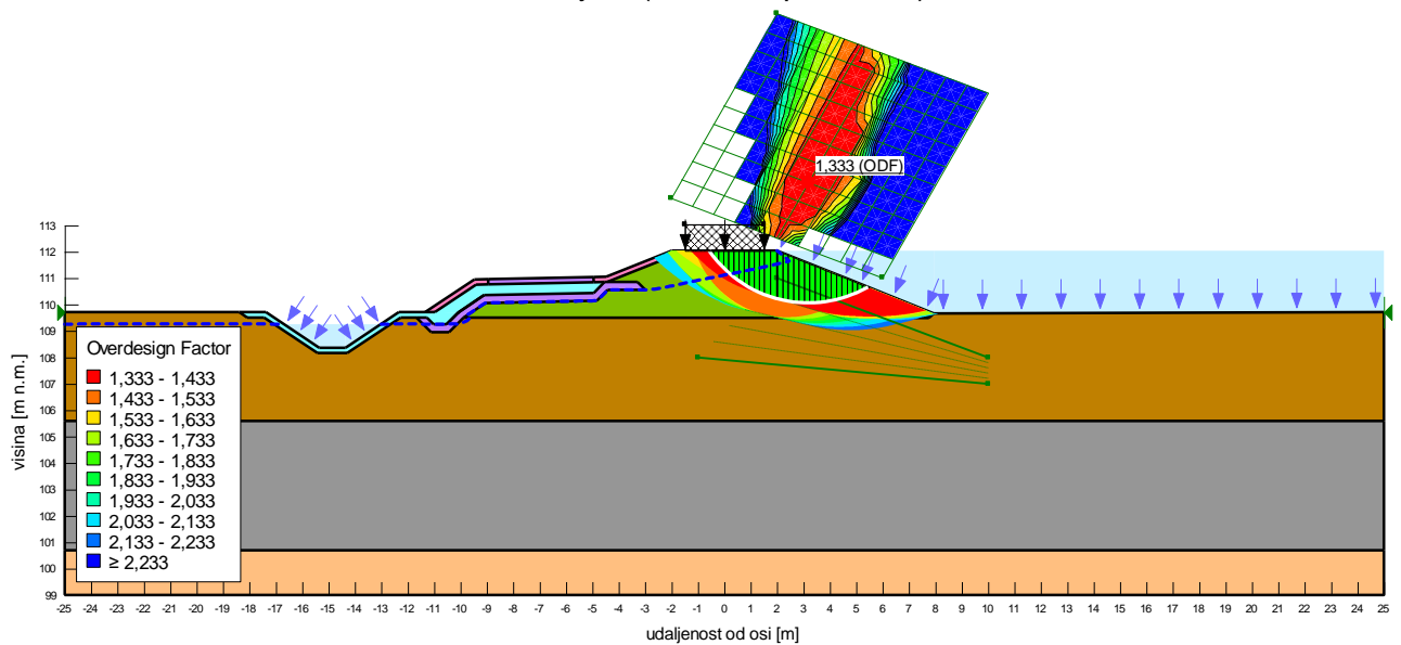
Slika 4.1.41: Situacija 4, uzvodni pokos, drenirano stanje
