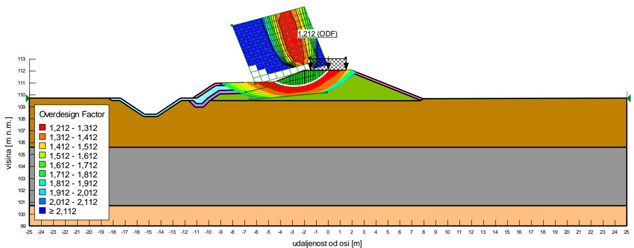
Slika 4.1.33: Situacija 1, nizvodni pokos, drenirano stanje
