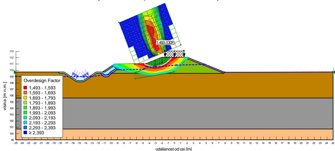
Slika 4.1.27: Situacija 5, nizvodni pokos, drenirano stanje
