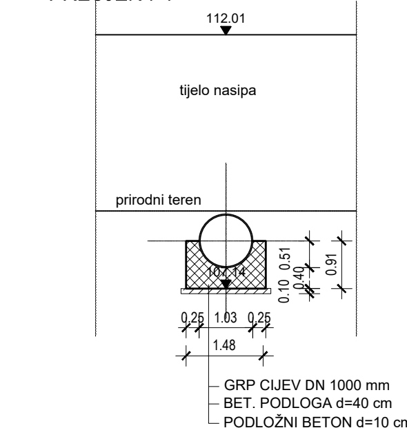
PRESJEK 7-7
