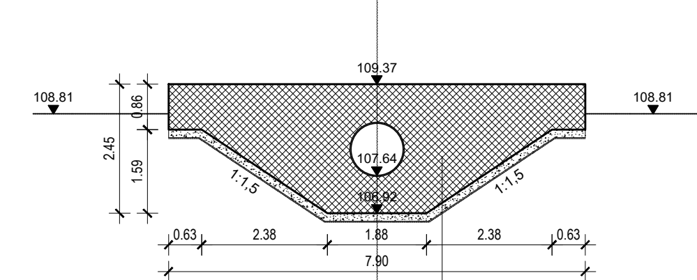
PRESJEK 9-9
