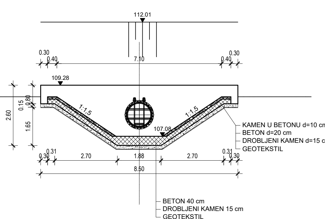
PRESJEK 4-4
