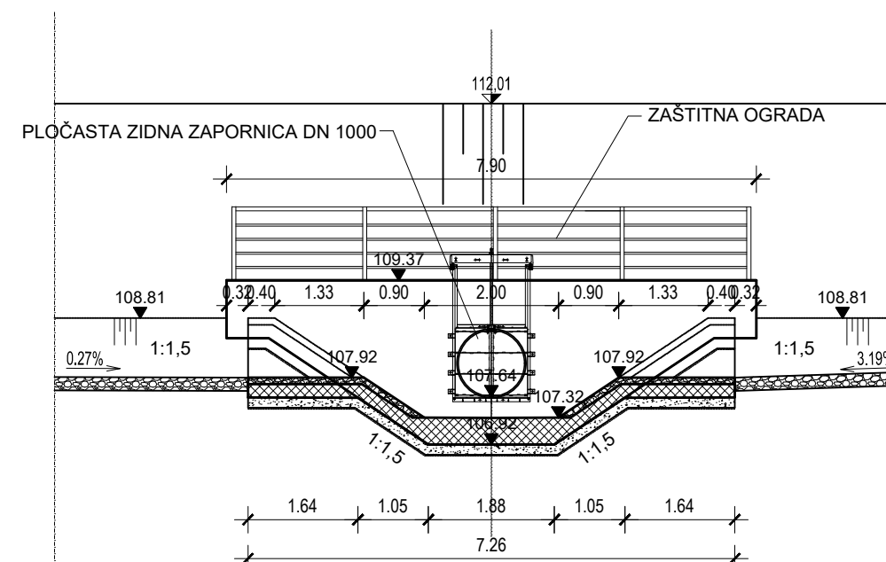
PRESJEK 10-10
