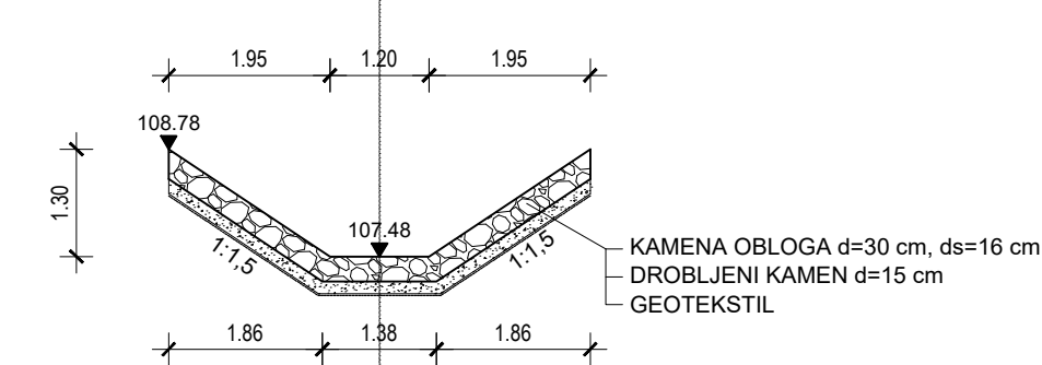
PRESJEK 1-1
