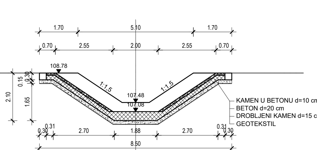
PRESJEK 3-3
