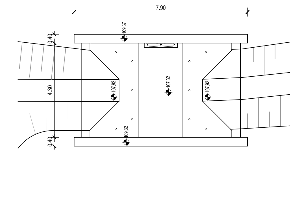
PRESJEK 10-10
