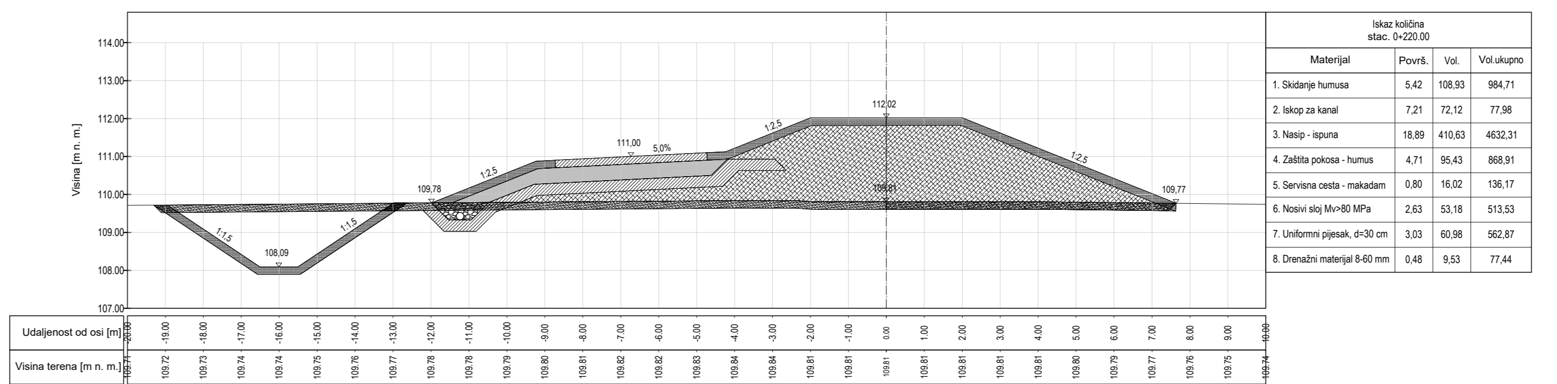
PR-12 0+220.00
