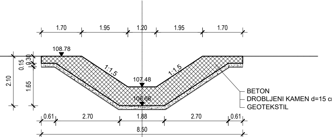
PRESJEK 2-2
