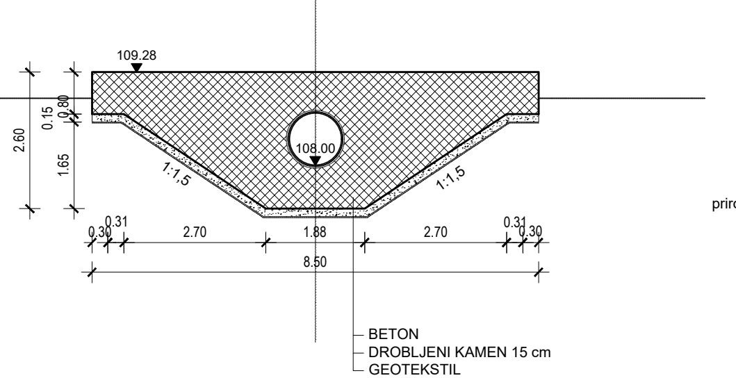
PRESJEK 5-5
