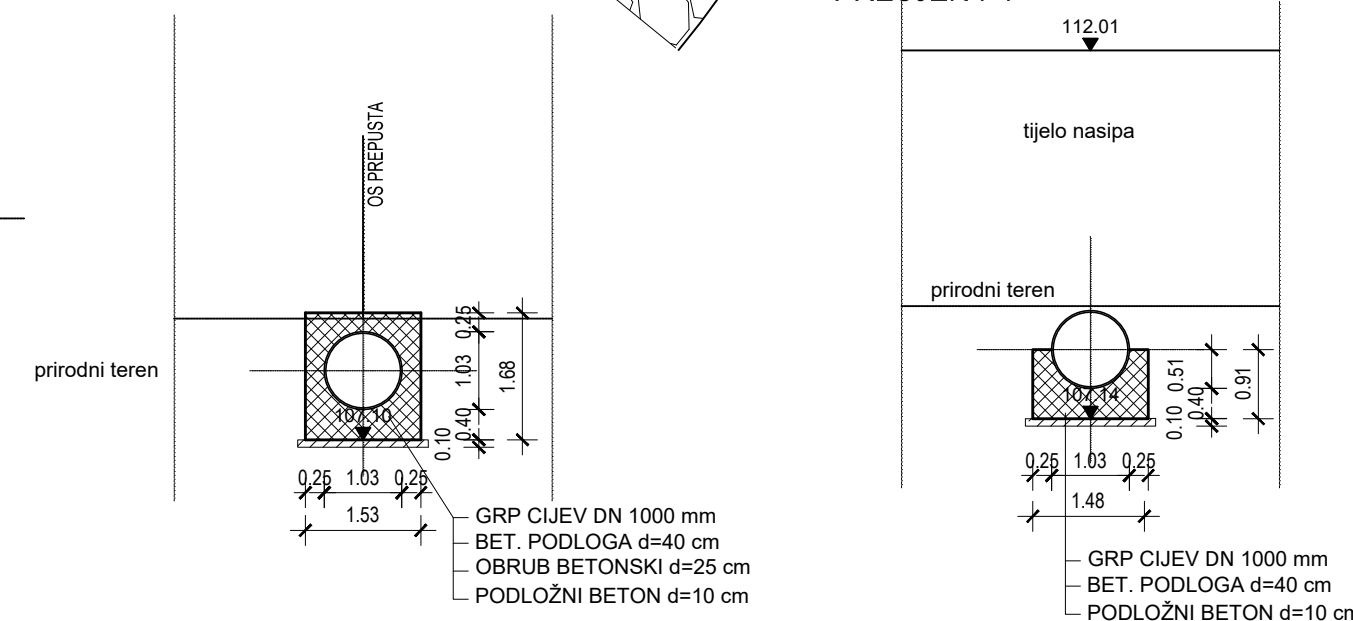
PRESJEK 6-6
