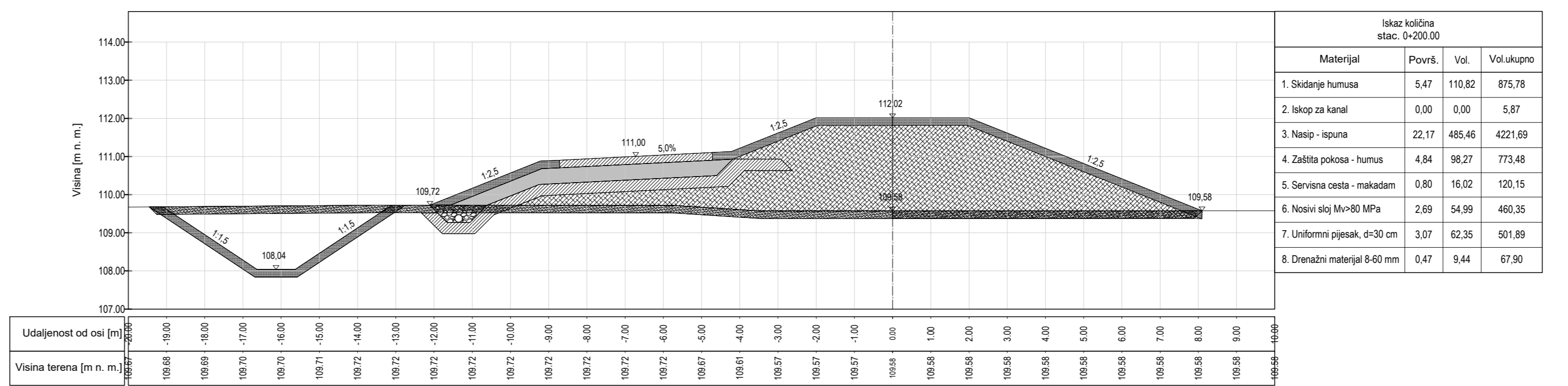
PR-11 0+200.00
