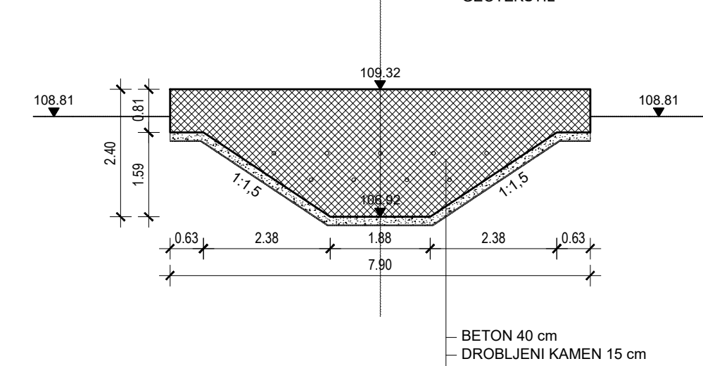
PRESJEK 11-11
