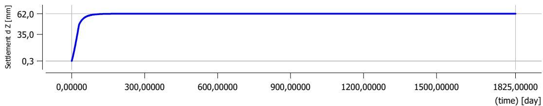
Slika 3-37: Model 3 – slijeganje krune nasipa u osi tokom vremena.
