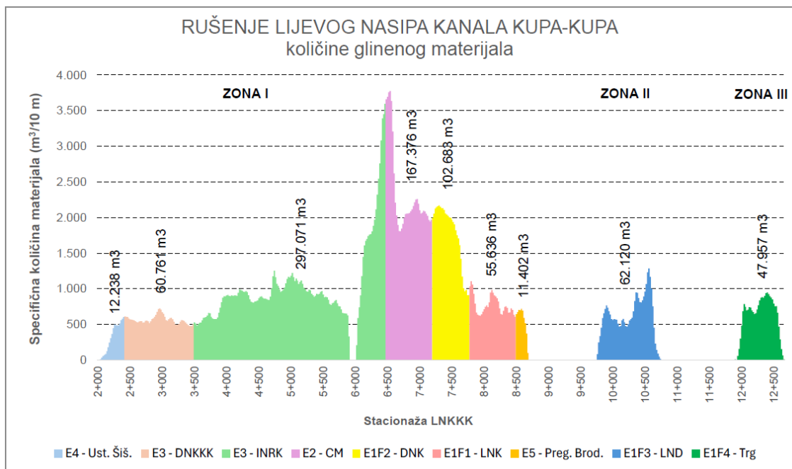
Slika 2-9: Raspodjela glinenog materijala dobivenog rušenjem lijevog nasipa kanala Kupa-Kupa po etapama/fazama
