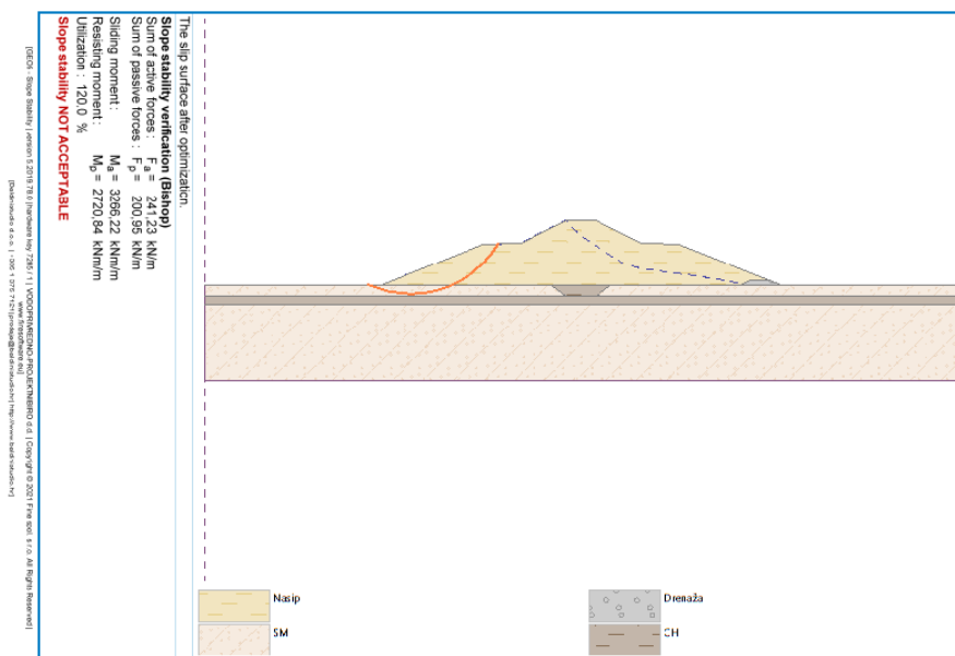
Slika 3-14: Model 2- Klizna ploha za projektnu situaciju 3.
