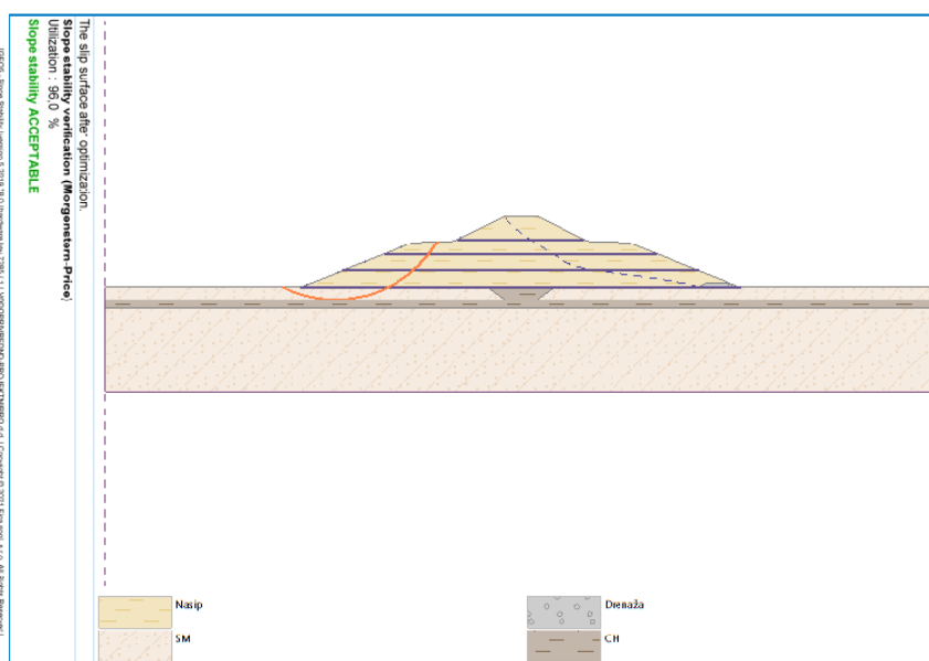
Slika 3-15: Model 2- Klizna ploha za projektnu situaciju 4.
