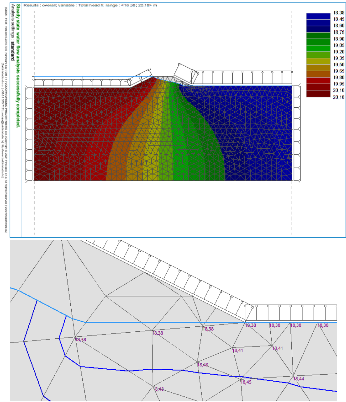
Slika 3-8: Rezultati analize procjeđivanja (iznos tlakova): Model 4: KM 3+486,00 – Projektna situacija 2.
