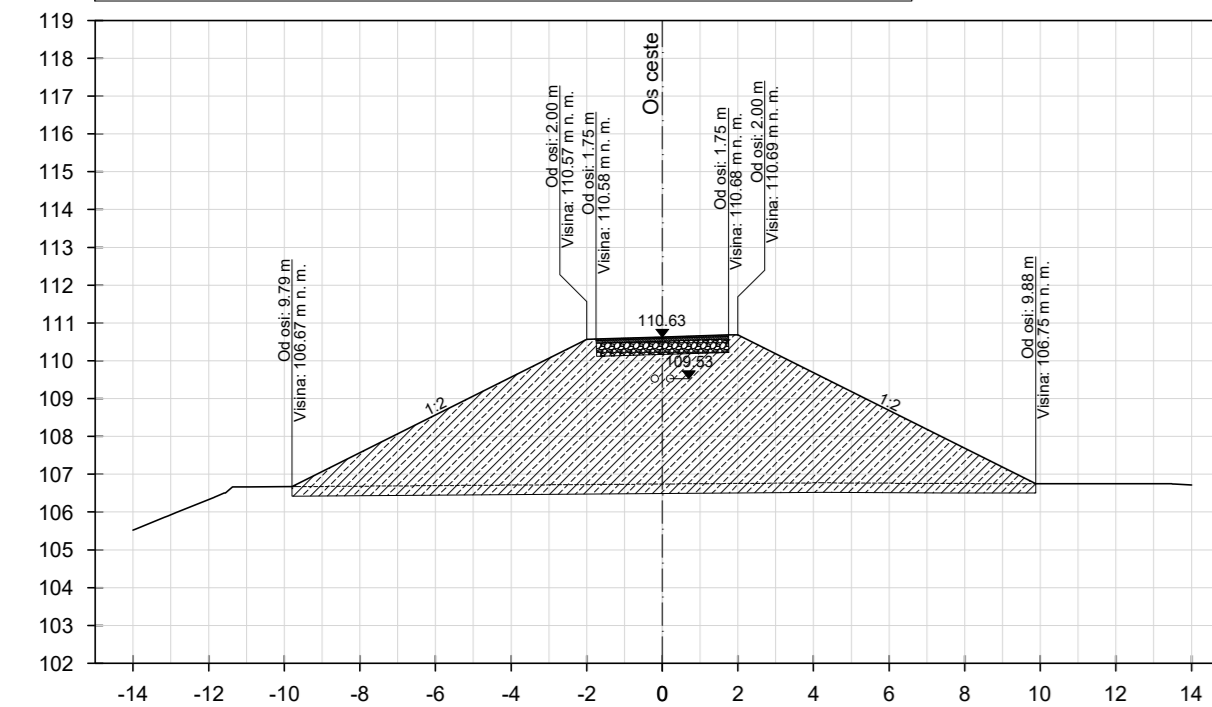
POPREČNI PRESJEK - P20 - stac. km 0+380.00
