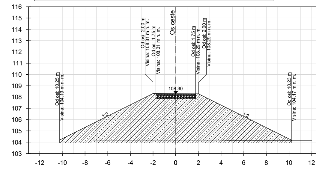
POPREČNI PRESJEK - S4 - stac. km 0+060.00
