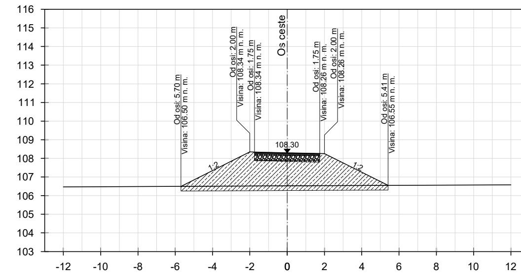
POPREČNI PRESJEK - S3 - stac. km 0+040.00
