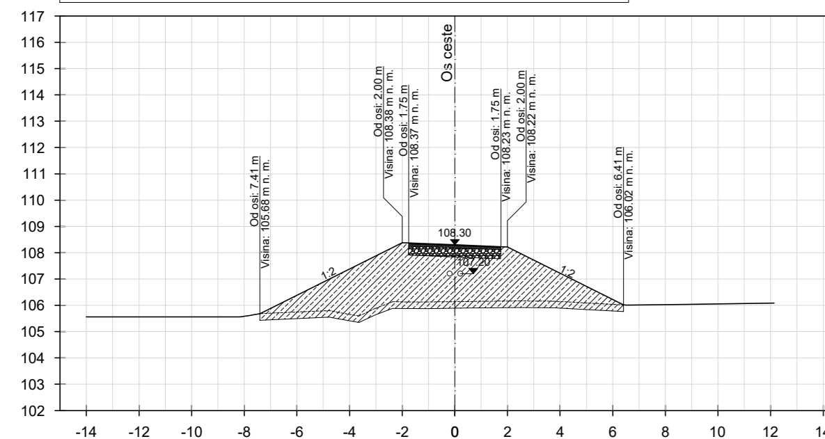
POPREČNI PRESJEK - P05 - stac. km 0+080.00
