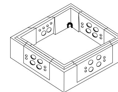
UVODNA PLOČA TIP A (3 kom)
