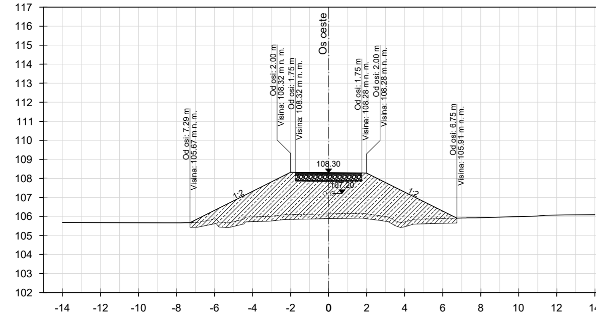
POPREČNI PRESJEK - P02 - stac. km 0+020.00
