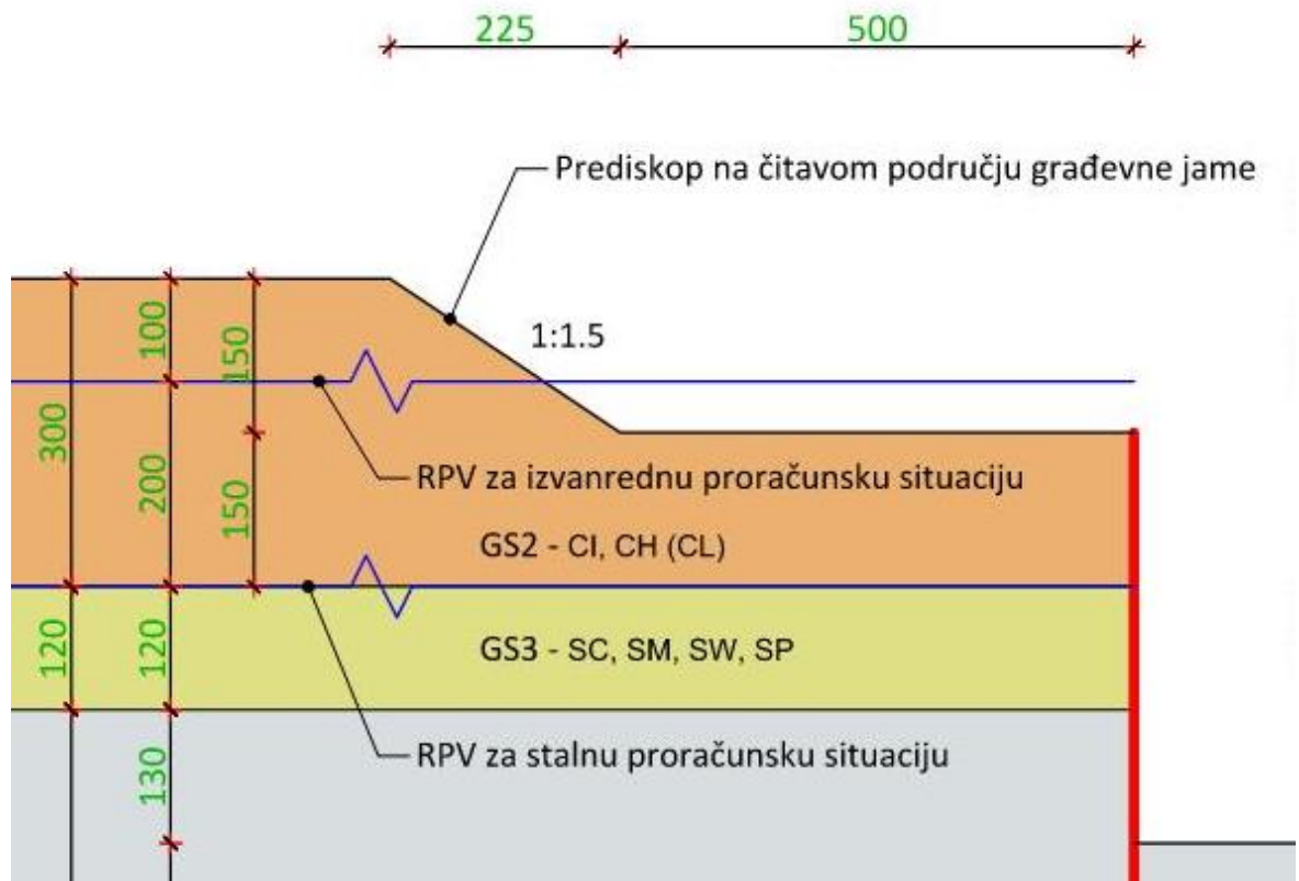
Slika 5.5-1 Pojednostavljeni prikaz proračunskog modela
