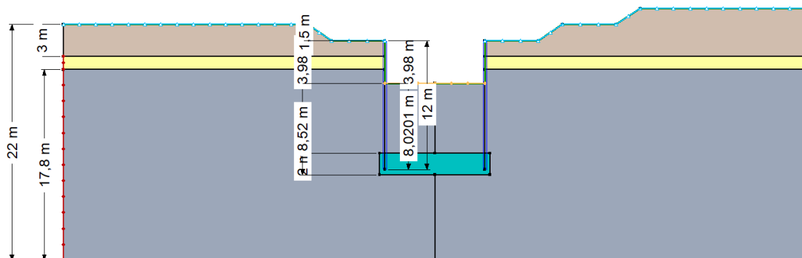
Slika 5.6-7 Prikaz modela poprečnog presjeka 1-1
