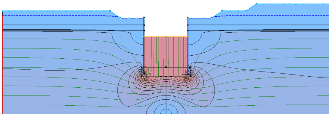
Slika 5.6-22 Prikaz modela poprečnog presjeka 1-1
