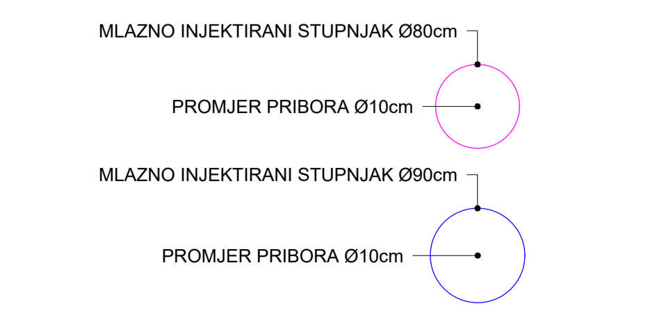
STUPNJACI ZA POPUNJAVANJE OTVORA RASTERA STUPNJAKA Ø90 I Ø120
