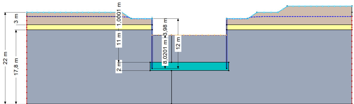
Slika 5.6-25 Prikaz rezultata procjeđivanja poprečnog presjeka 2-2
