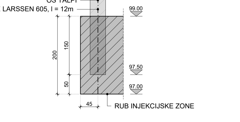
DETALJ SPOJA MLAZNO INJEKTIRANIH STUPNJAKA I TALPI MJ 1:50
