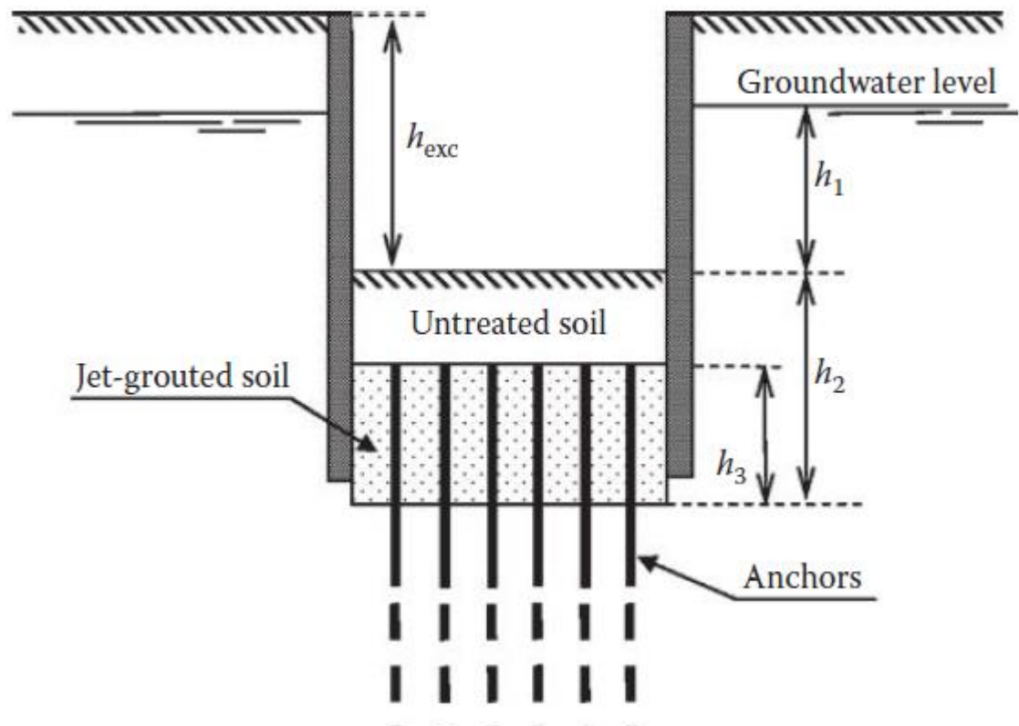
Slika 5.4-1 Shematski prikaz brtvenog sloja od mlaznoinjektiranih stupnjaka uzimajući u obzir moguće postojanje sidara i neojačanog tla na vrhu stupnjaka
