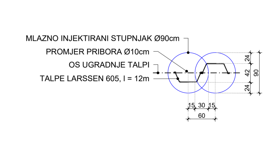
HEMA UGRADNJE MLAZNO INJEKTIRANIOG STUPNJAKA Ø90cm MJ 1:50
