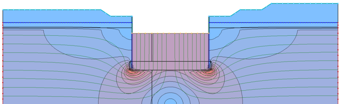
Slika 5.6-10 Prikaz rezultata procjeđivanja poprečnog presjeka 2-2
