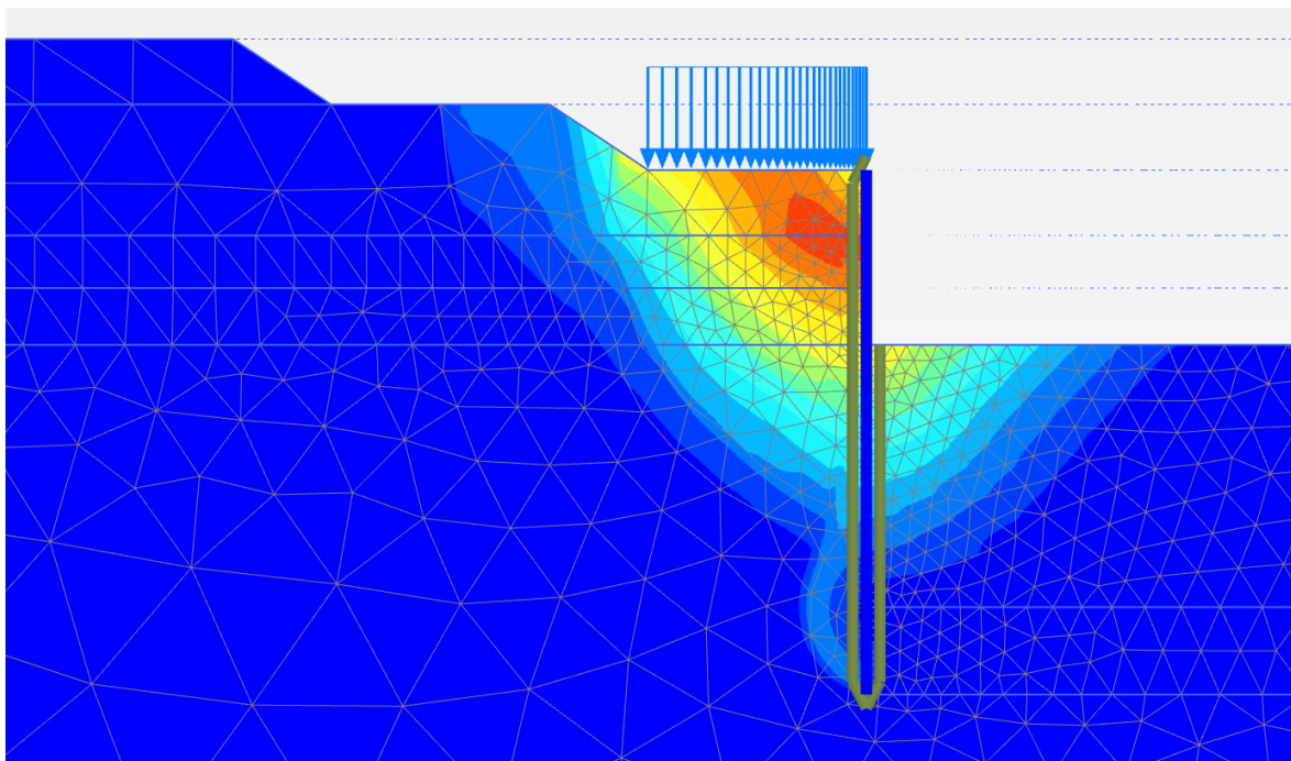
Slika 5.3-13 \phi -c analiza - prikaz mehanizma sloma (prikaz u konačnoj fazi – faza 6); postignuti F_s=1.502
