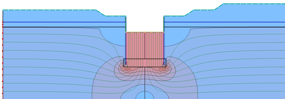
Slika 5.6-7 Prikaz modela poprečnog presjeka 1-1
