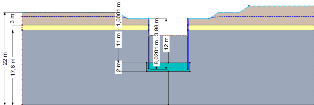
Slika 5.6-22 Prikaz modela poprečnog presjeka 1-1
