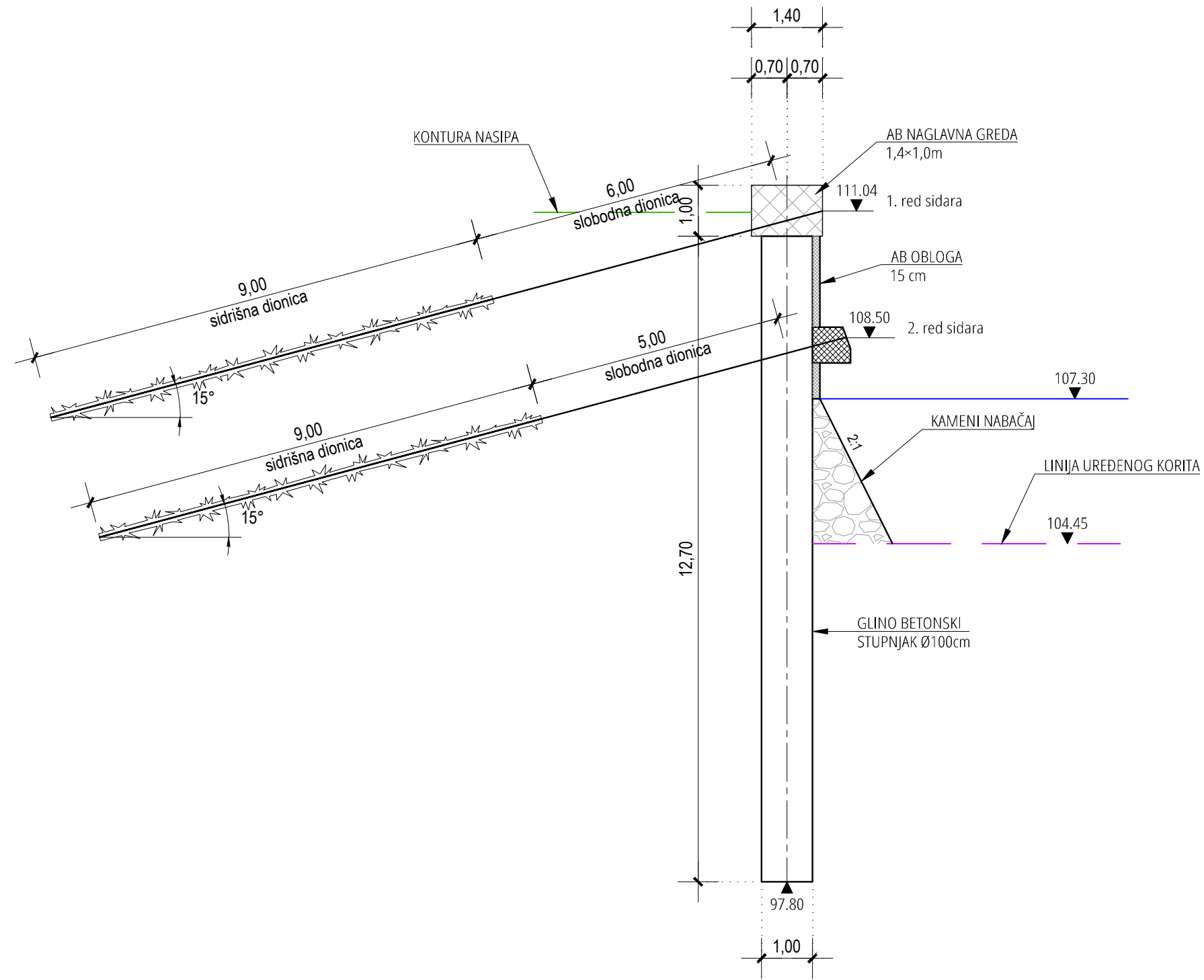
PILOTNA STIJENA PS3 POPREČNI PRESJEK 5-5
