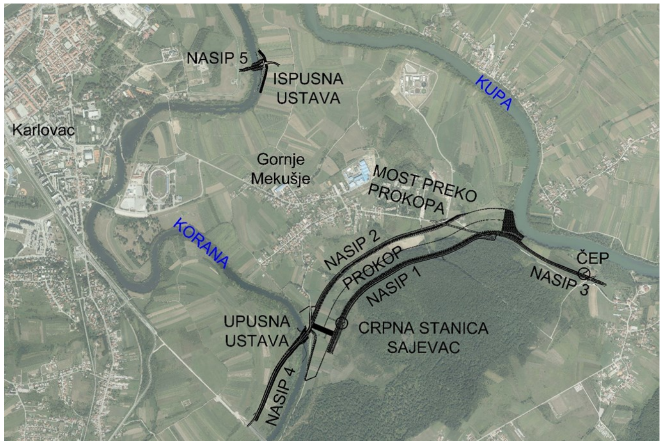
Slika 1-3: Građevine zahvata
