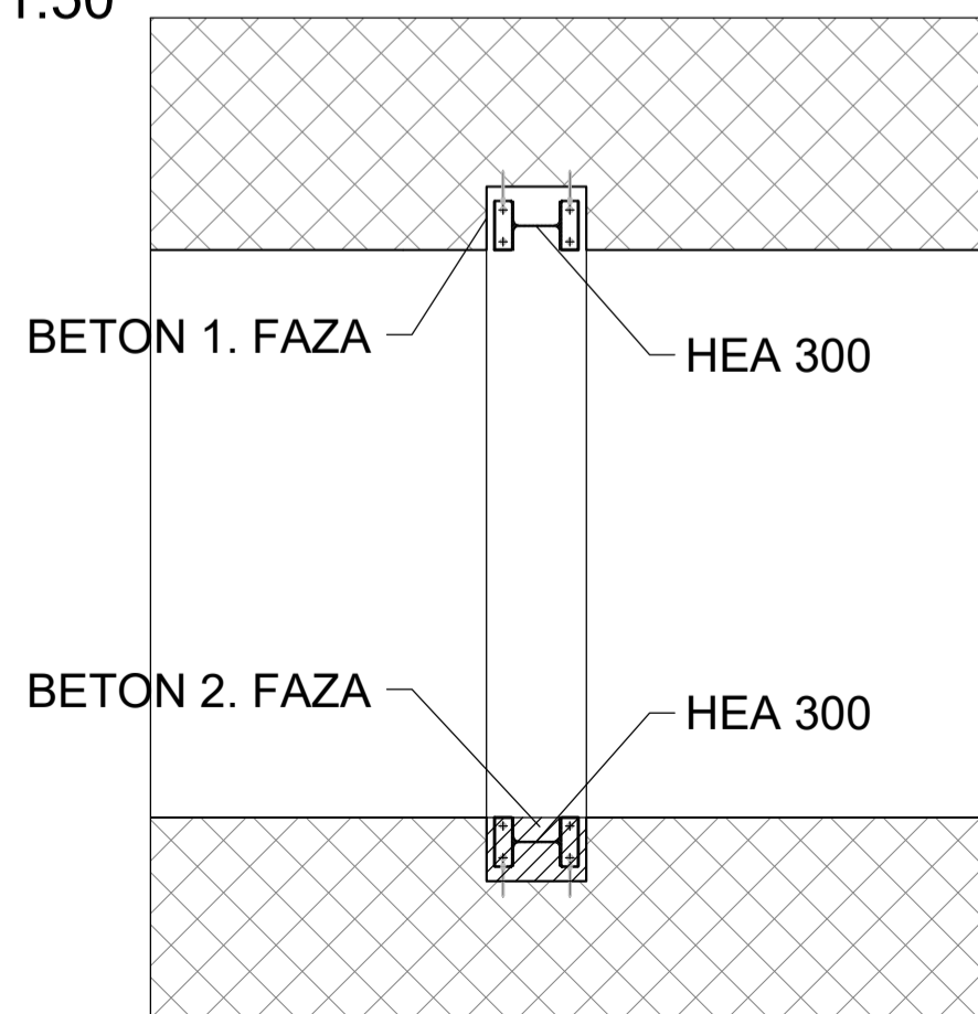
DETALJ 1 MJ 1:50
