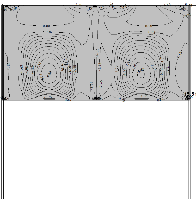
Okvir: V_2 Utjecaji u ploči: max M_y = 0.00 / min M_y = -15.51 kNm/m
