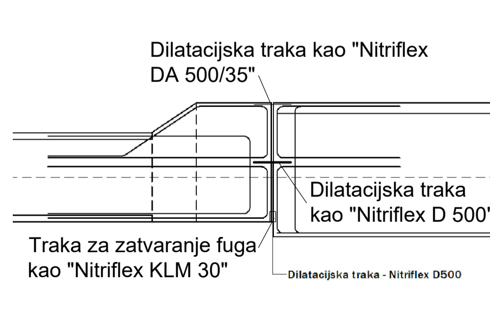
DETALJ 2 MJ 1:50
