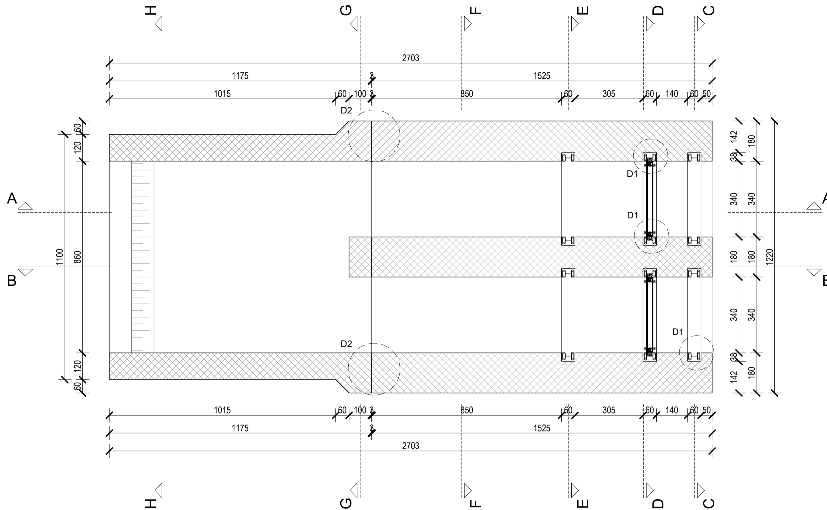
DETALJ 1 MJ 1:50
