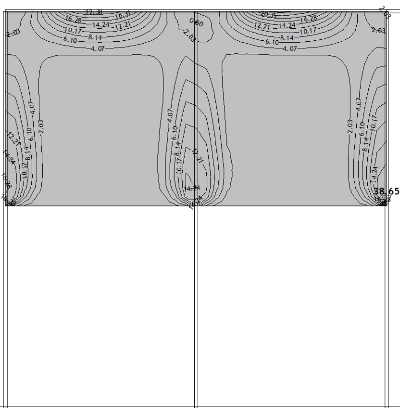
Okvir: V_2 Utjecaji u ploči: max M_y = 38.65 / min M_y = 0.00 kNm/m
