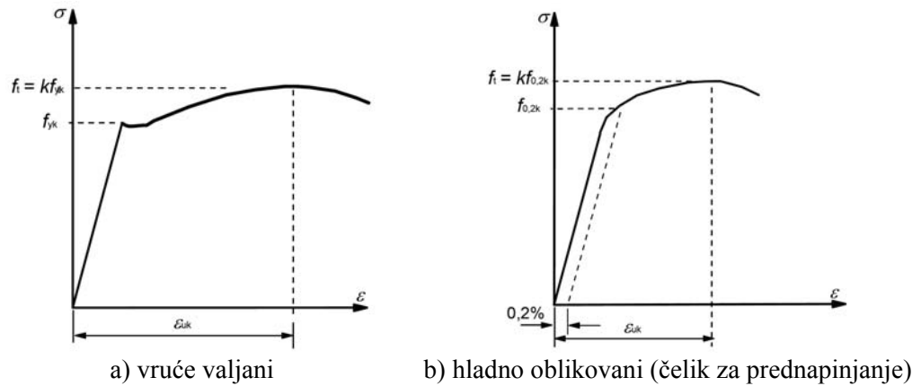
Slika 6-00.2.2-2 Dijagrami napon-deformacija tipičnog čelika za armiranje
