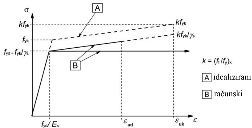
Slika 6-00.2.2-3 Idealni i računski dijagrami napon-deformacija čelika za armaturu (za vlak i tlak)
