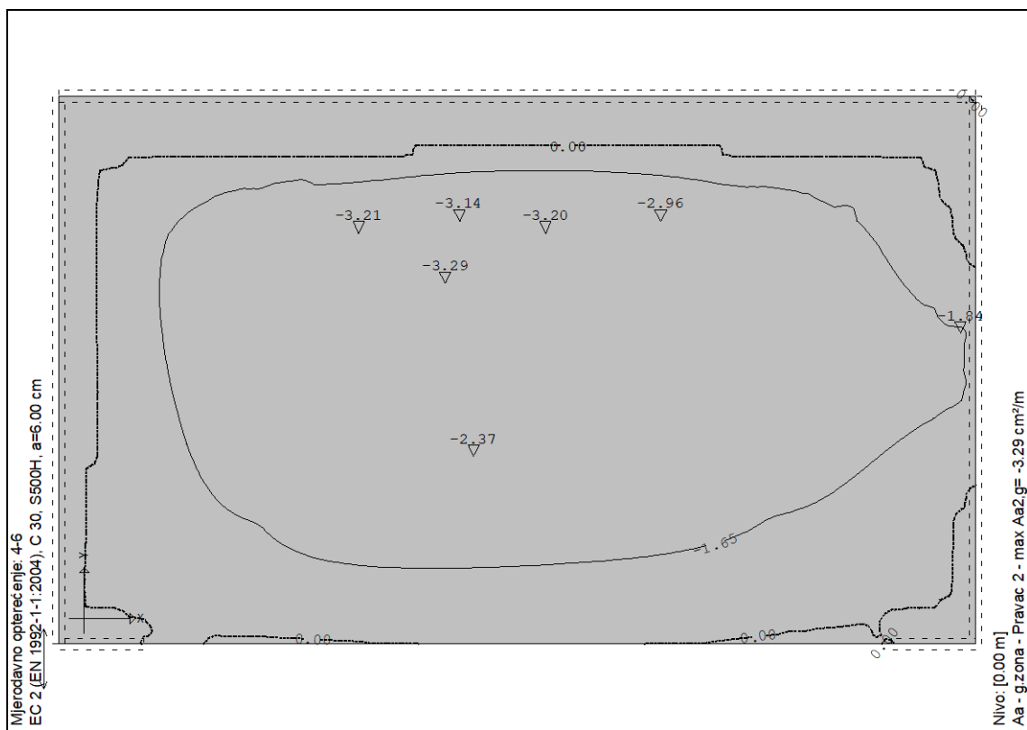
Slika: Proračunska armatura temeljne ploče
